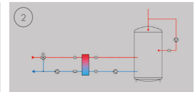
Beimischung primär
