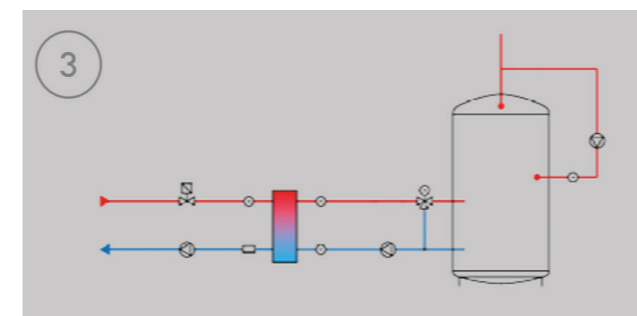
Beimischung sekundär
