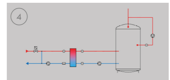
Einspritzung
